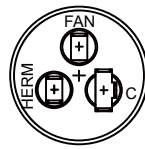
e) AMP250#插件(1+2+长3)
