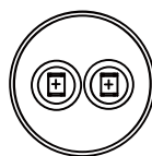
b) AMP250#插片(2+2)
